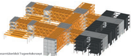
Gesamtüberblick Tragwerkskonzept
