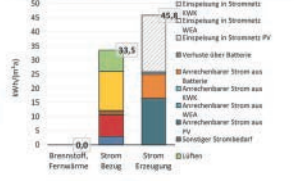
Endenergiebilanz
