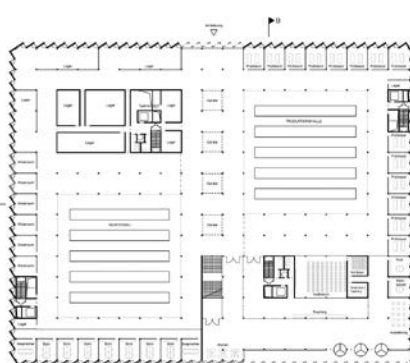
ERDGESCHOSS 1.500
