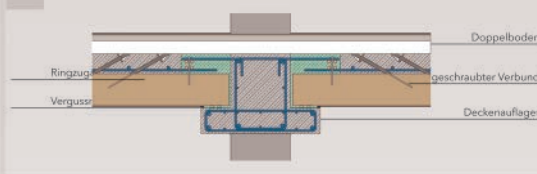
Leitdetail Anschluss
