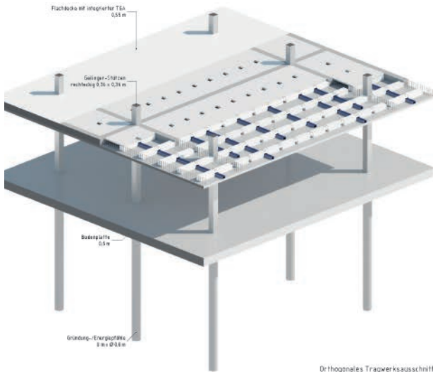
Orthogonales Tragwerksausschnitt
