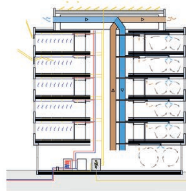
Energiekonzept im Sommer
