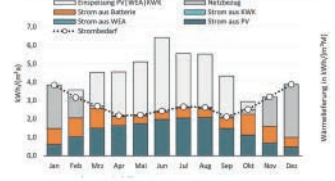
Strombilanz PV & KWK & WEA
