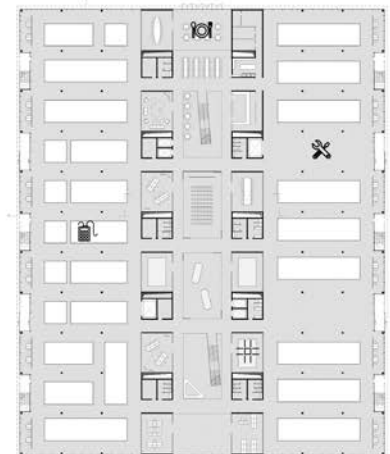
Grundriss EG M 1:500
