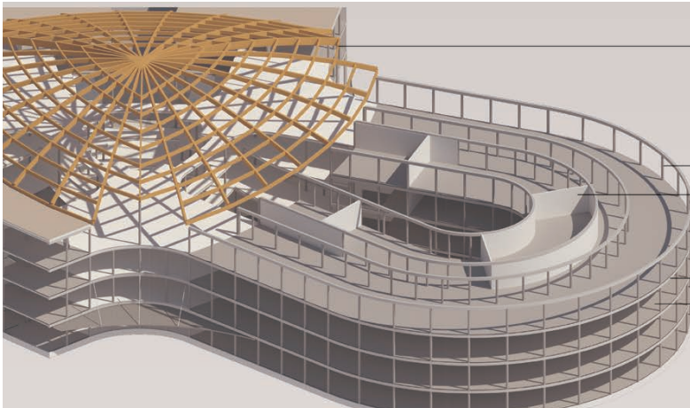
Bauablauf der Brettschichtholz-Kuppel im freien Vorbau
