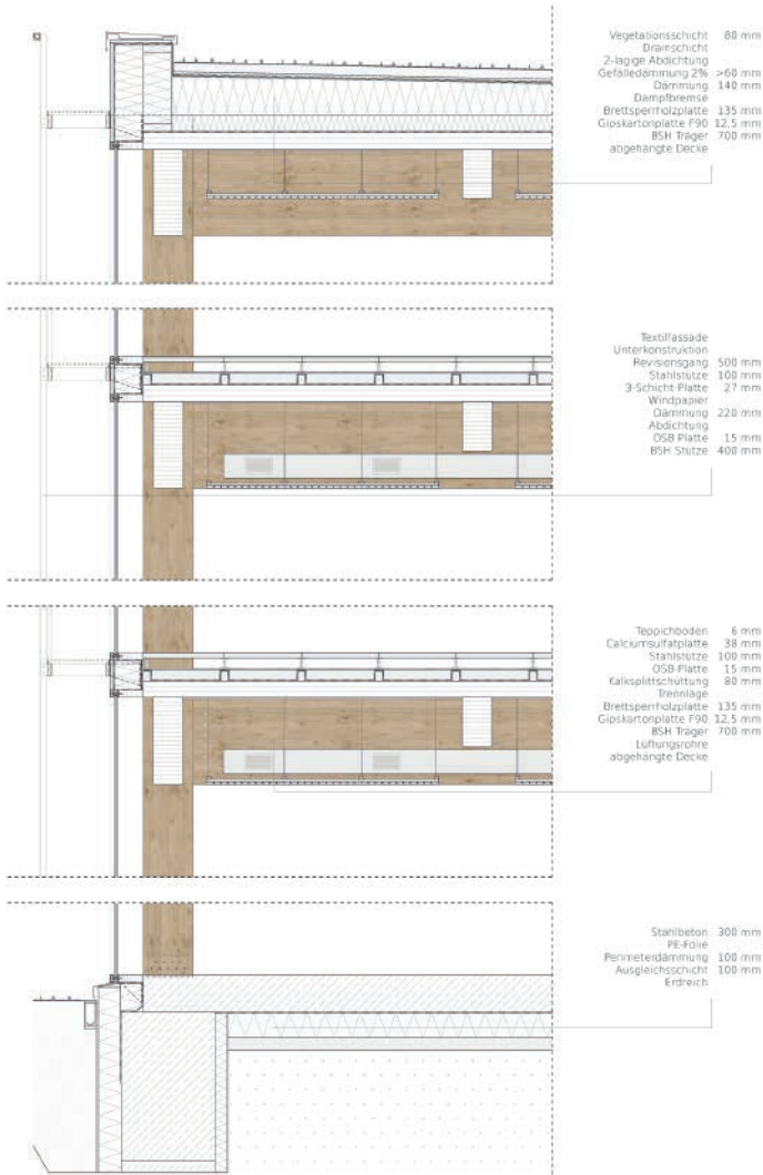
Fassadenschnitt M 1:20
