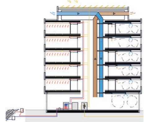
Energiekonzept im Winter
