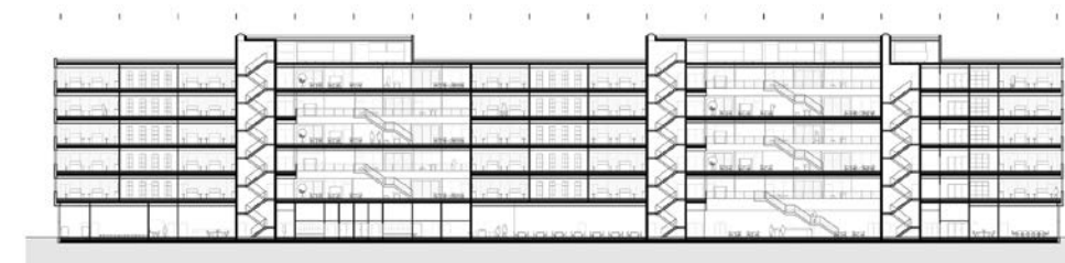
Längsschnitt Bürogebäude
