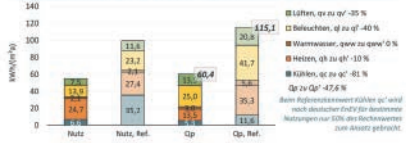
Energiebedarf Original- und Referenzgebäude
