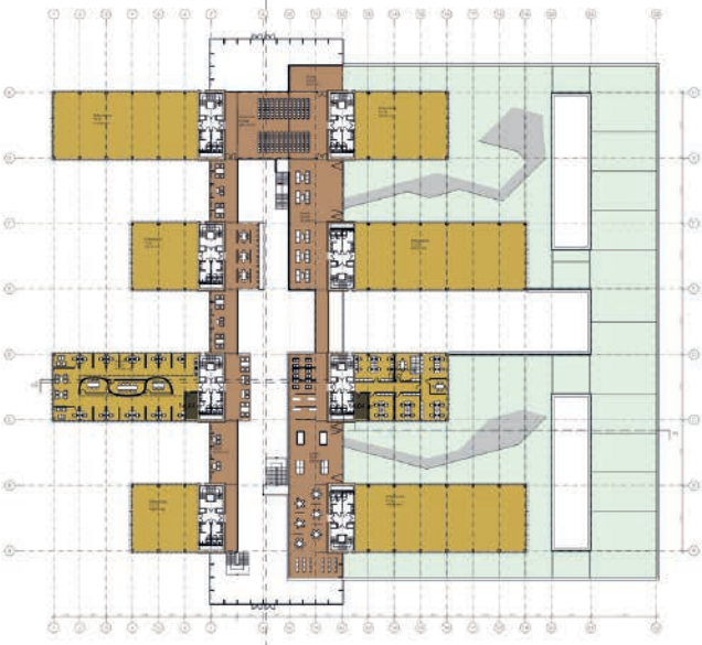
Grundriss OG2 1:500
